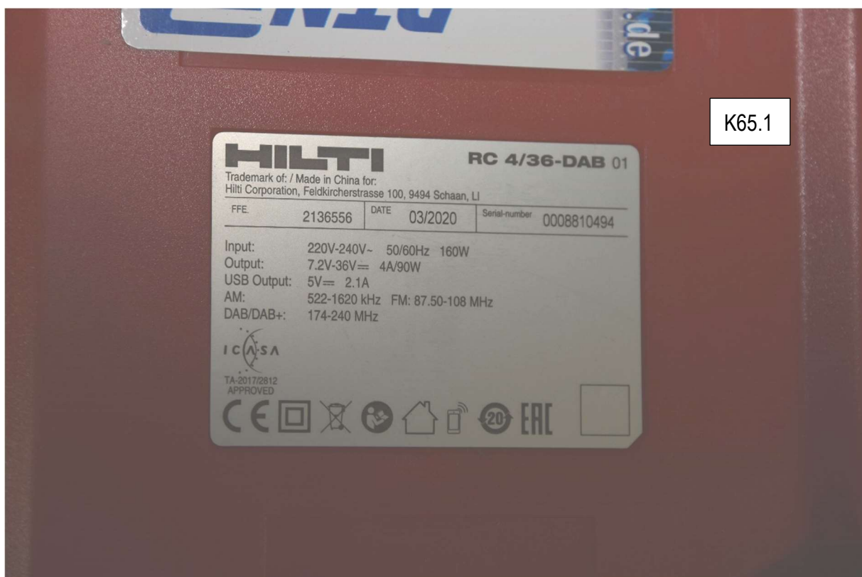
Detail Baustellenradio
